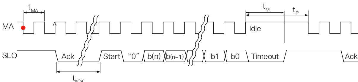
时序图:
