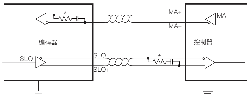
BISS-C 电气连接图:
